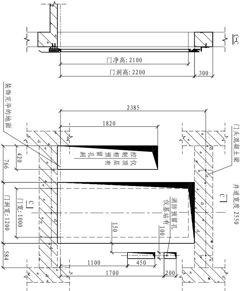
厅门正面图
